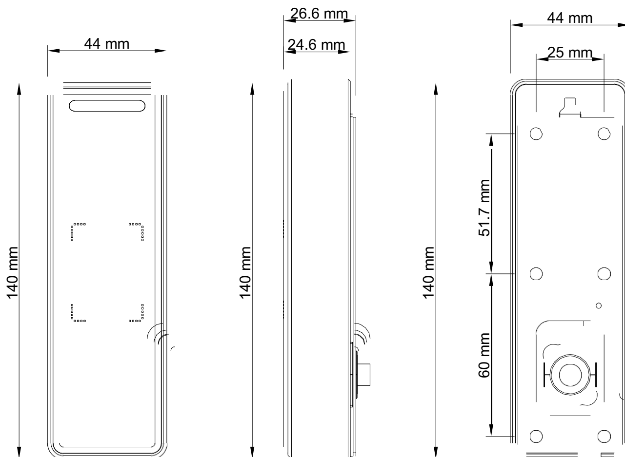
Pogled sprijeda
