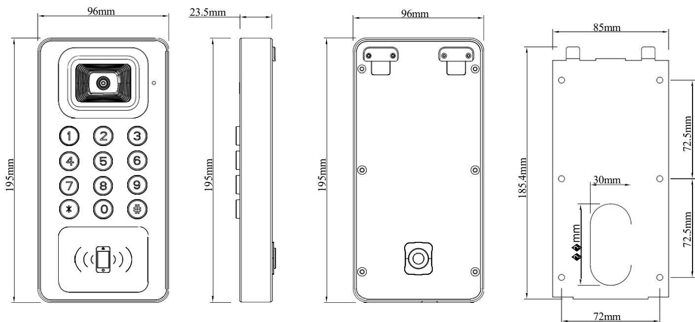
Pogled sprijeda
